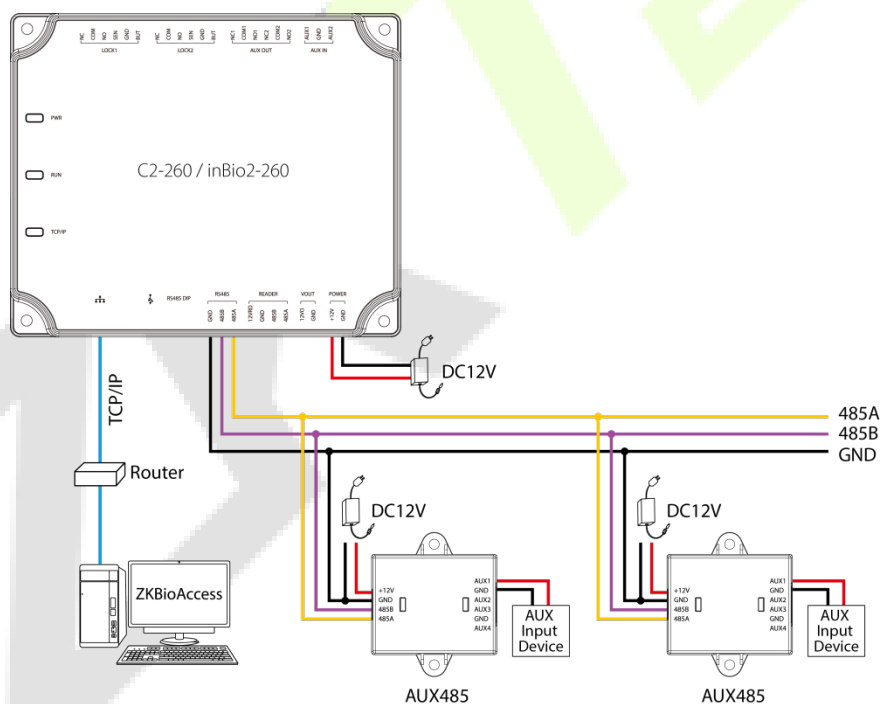
Подключение к AUX485 с помощью RS485
